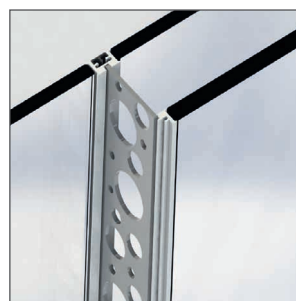
3. Sortir le premier vitrage de la lisse
